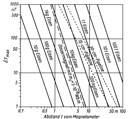
Abb. A-3.1-18 Nomogramm zur Abschätzung der maximalen Störwirkung dF_{max} von Eisenobjekten mit mc = 5 \cdot 4 \pi \cdot 10^{-8} \text{ Wb m je Kilogramm} nach BREINER (1973), entnommen aus KNÖDEL et al. 1997. Beachte: dF_{max} kann sich in Abhängigkeit von der Härte des Eisens, der Inklination sowie der Lage des Vektors der remanenten Magnetisierung um den Faktor 5 ändern.
