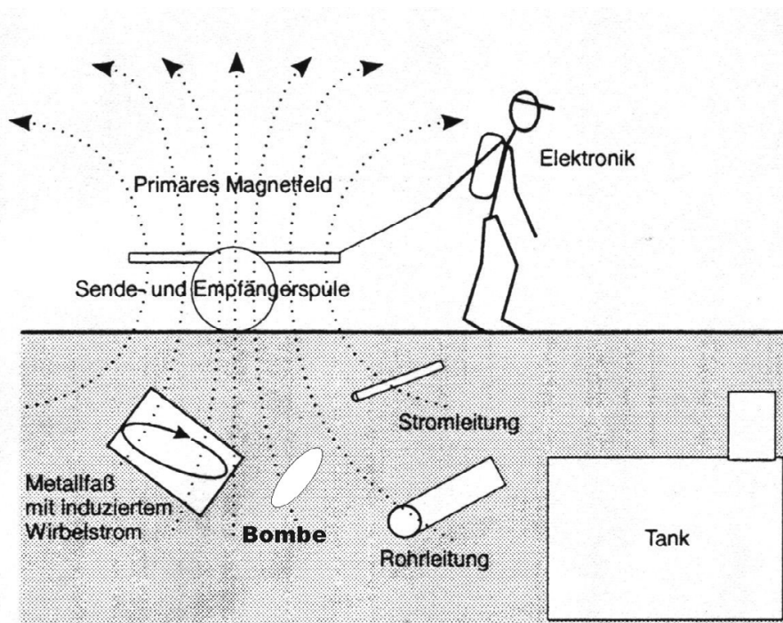
Abb. A-3.1-27 Schematische Funktionsweise und typische Untersuchungsobjekte des tiefeindringenden Metalldetektors (entnommen und modifiziert aus KNÖDEL et al., 1997)
