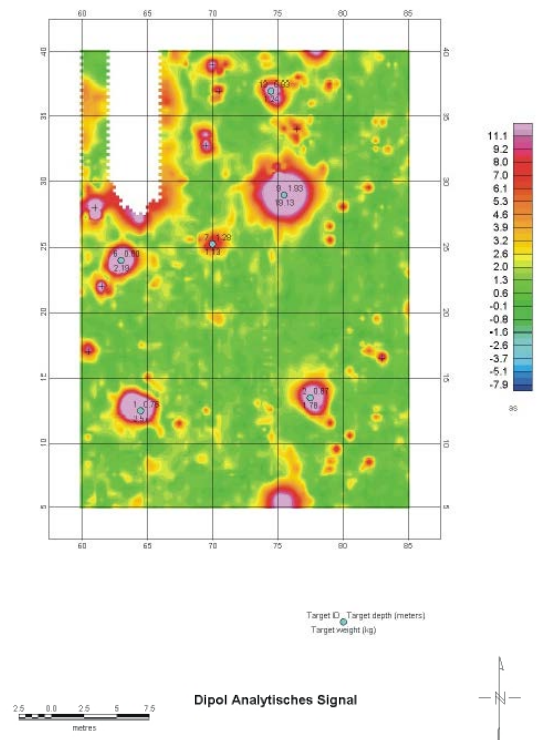
Abb. A-3.1-17 „Analytisches Signal mit Tiefenbestimmung“ für die Felddaten von Abbildung A-3.1-13
