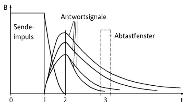
Abb. A-3.1-25 Signale beim Pulsinduktionsverfahren
