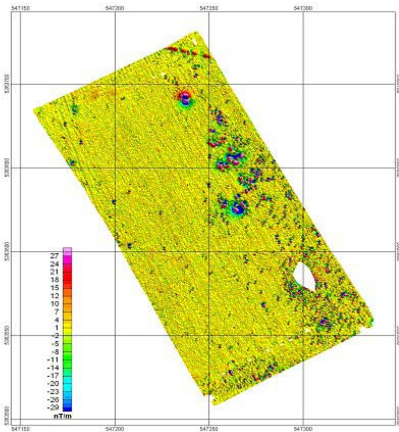
Abb. A-3.2-3 Ungleichmäßige Verteilung der Störkörper in einem 2 ha großen Testfeld
