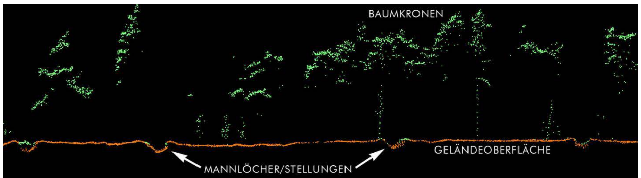
Abb. 2.3-3 Querschnitt durch eine Punktwolke (Quelle: Daten: NLBL, Darstellung: Luftbilddatenbank Dr. Carls GmbH)
