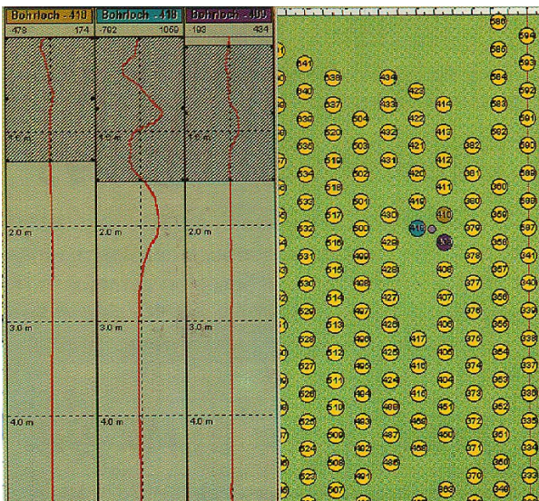
Abb. A-3.1-10 Beispiel eines Bohrlochfeldes inkl. einer Störkörperortung mit Magnetik
